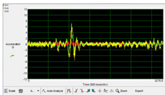
バイク荷台の振動波形
