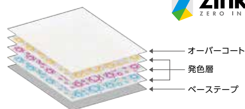
ラベル断面図
