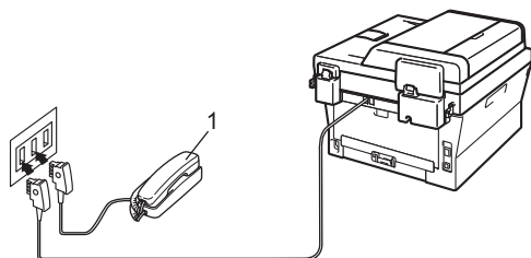
1 Externes Telefon
