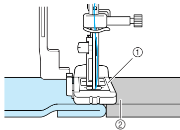
① Прижимная лапка ② Толстые материалы
