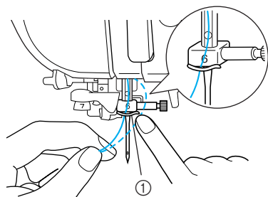
① Нитенаправитель игловодителя
