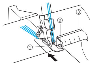
① 压脚 ② 上切刀 ③ 缝边导线
