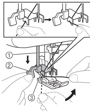
① Suport pentru ac ② Pârghie dispozitiv de înfilare ac ③ Conducător de fir
