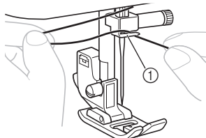
1 Conducătorul de fir de pe tija de fixare a acului
