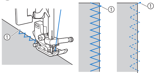
① 落针点
