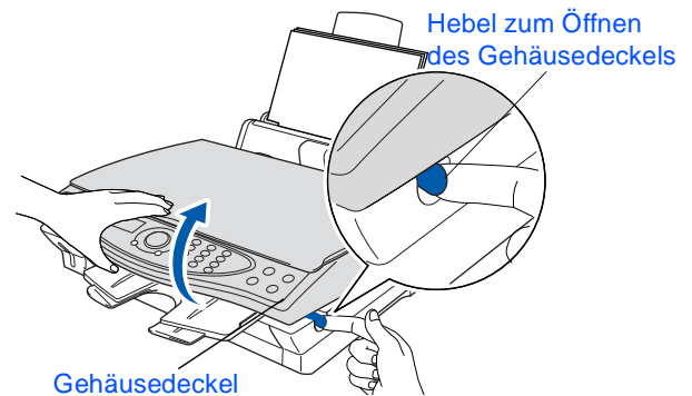
Gehäusedeckel
