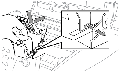
Druckkopfschutz befestigen
