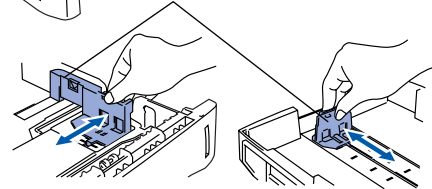
Ontgrendeling papiergeleiders
