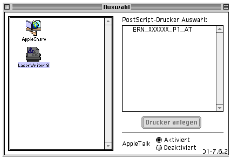
Abb. 2 Macintosh Auswahl
