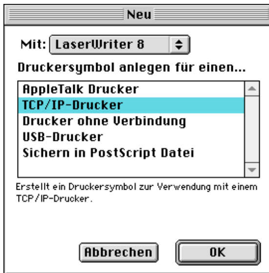
Abb. 3 TCP/IP-Druck wählen
