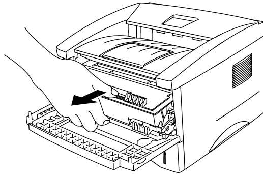
Fig. 3-13 Rimuovere il gruppo tamburo
