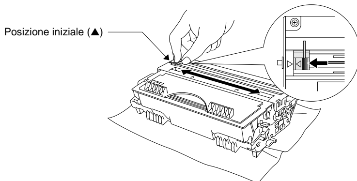
Fig. 3-10 Pulire il filo corona principale
