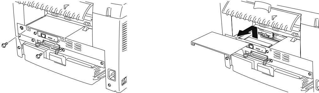
Fig. 2-3 Rimuovere il Controller PCB principale
