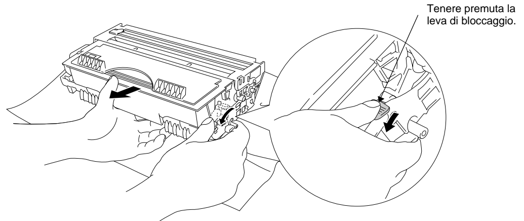
Fig. 3-4 Rimuovere la cartuccia di toner usata
