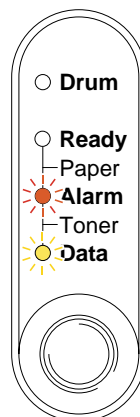
Fig. 3-1 Segnalazione di toner insufficiente
