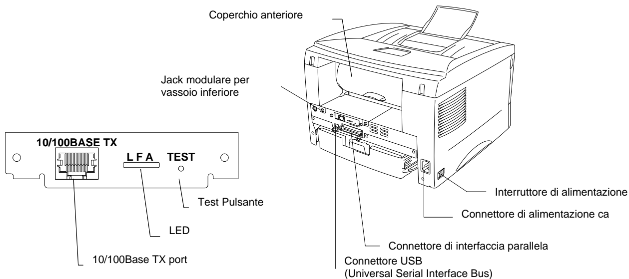
Fig. 1-3 Scheda di rete
