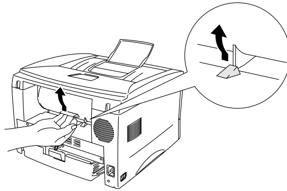
Fig. 1-17 Sollevare il coperchio posteriore
