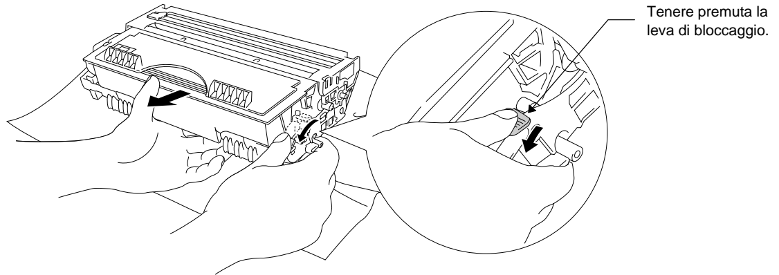
Fig. 3-15 Rimuovere la cartuccia di toner
