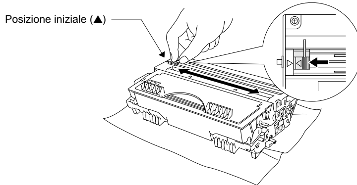
Fig. 3-22 Pulire il filo corona principale
