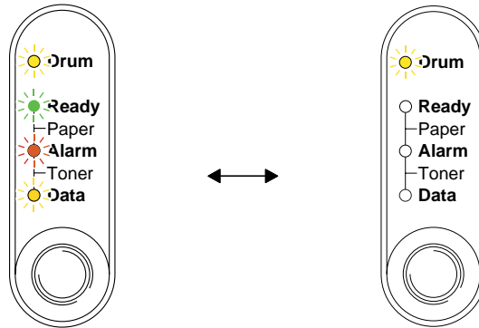
Fig. 4-2 Indicazioni visive dei LED per errore di funzionamento dell'unità di fusione
