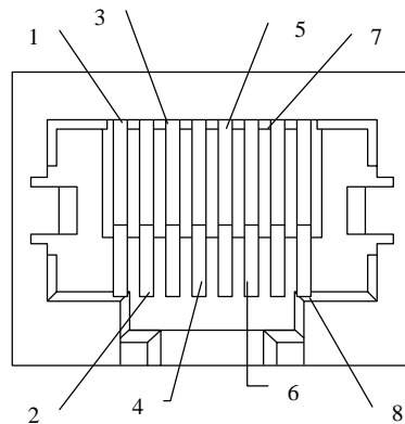
Fig. A-3 Porta 10/100Base TX
