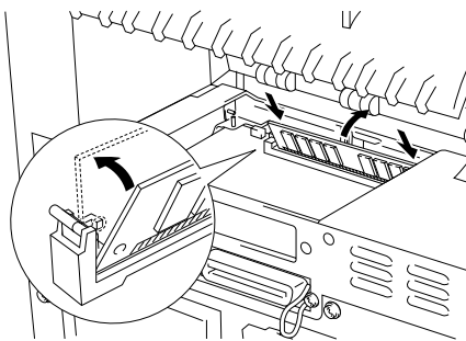
Fig. 2-5 Installare il modulo SIMM
