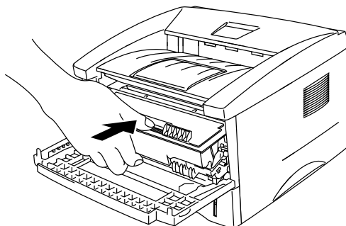
Fig. 3-17 Installare il nuovo gruppo tamburo
