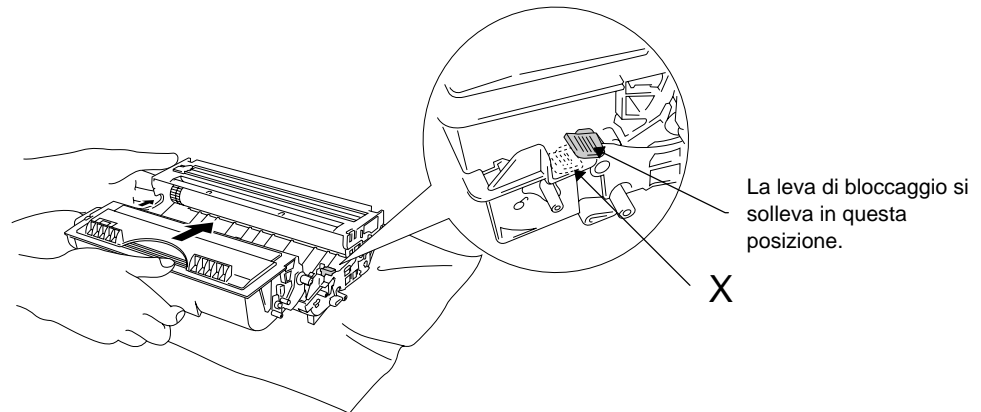
Fig. 3-9 Inserire la cartuccia di toner nel gruppo tamburo
