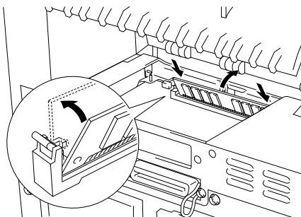
Fig. 2-5 Installera SIMM-modulen
