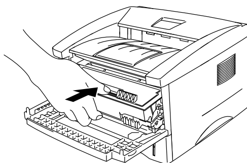
Fig. 3-17 Installera trumenheten
