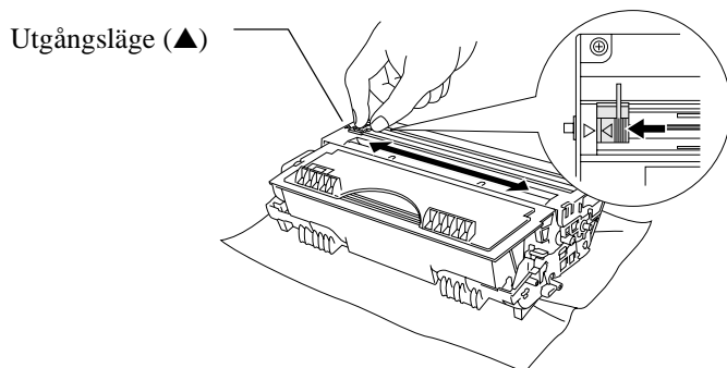
Fig. 3-22 Rengöra huvudkoronan
