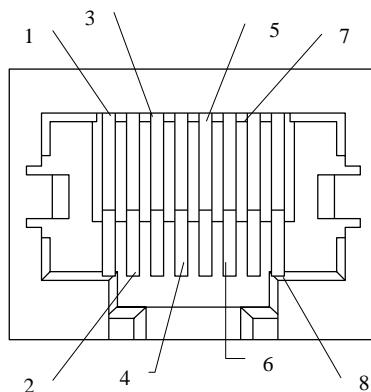
Fig. B-3 10/100 Bas TX Port
