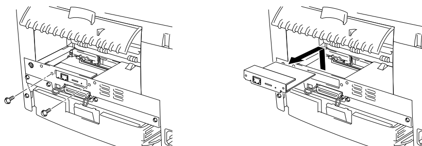
Fig. 2-4 Ta bort nätverkskortet
