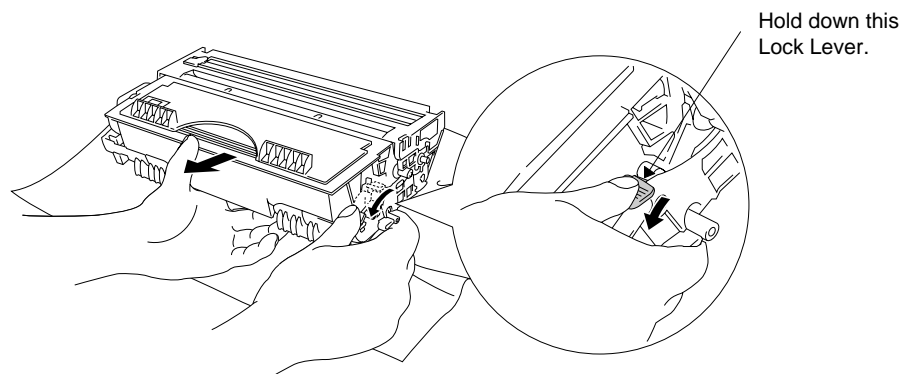
Fig. 3-4 Ta bort den gamla tonerkassetten
