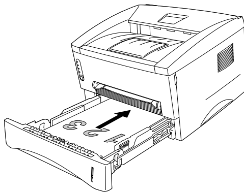
Fig. 1-19 Pappersriktning i papperskassetten
