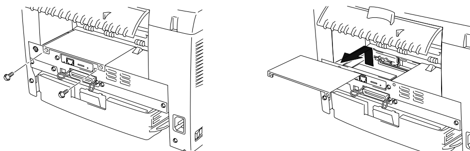
Fig. 2-3 Ta bort styrenheten
