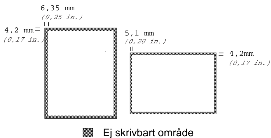
Fig. 1-7 Utskriftsområde
