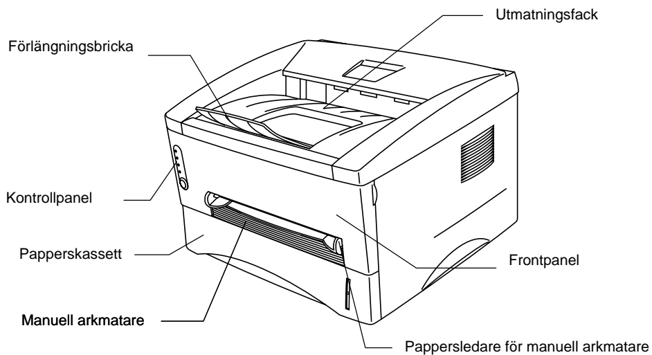
Fig. 1-2 Skrivaren sedd framifrån
