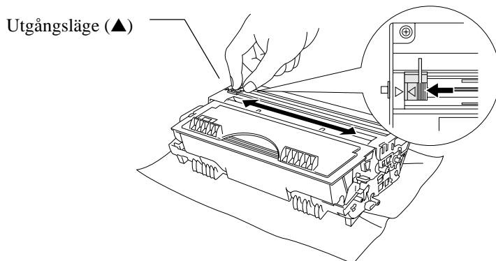
Fig. 3-10 Rengöra huvudkronan
