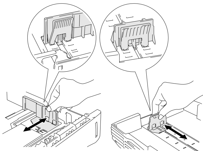
Fig. 1-9 Anpassa pappersledarna
