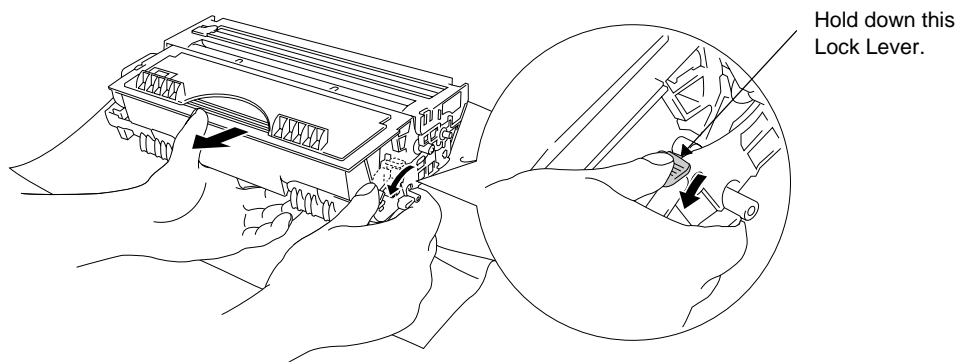
Fig. 3-15 Ta bort tonerkassetten
