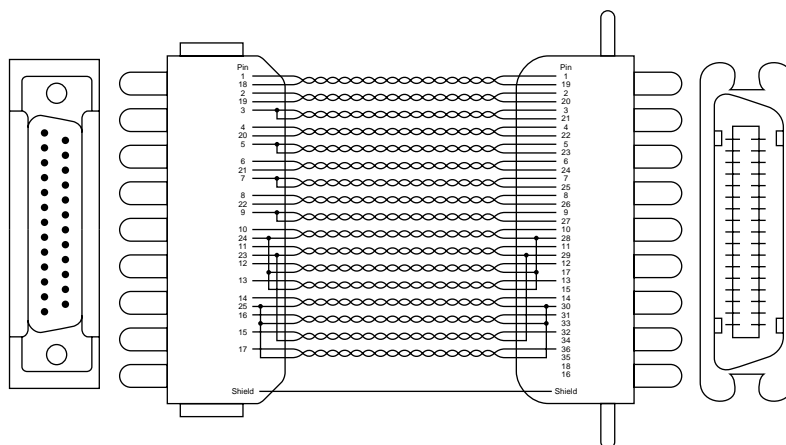
Fig. B-1 Parallell gränssnittskabel
