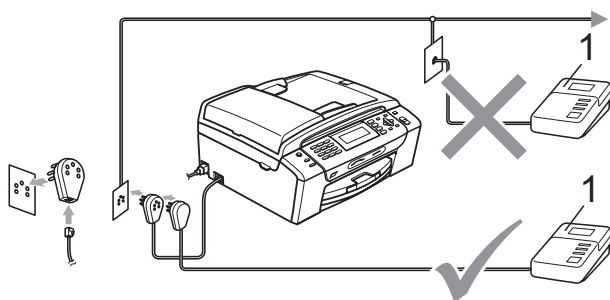
1 Antwoordapparaat
