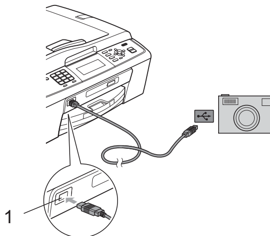
1 Interfaz directa de USB
