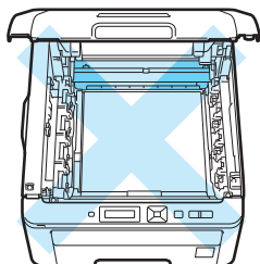
Interior del producto (Vista superior)
