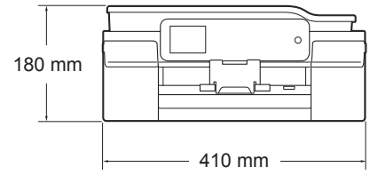
(DCP-J752DW)
