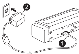
Tilslut lysnetadapteren.
