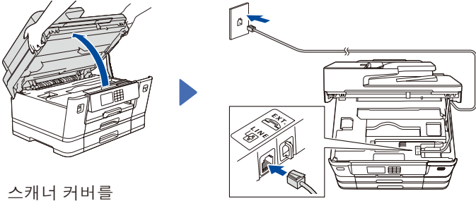
스캐너 커버를 들어올립니다.
