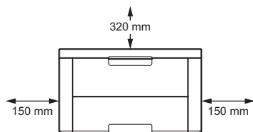
Visão frontal
