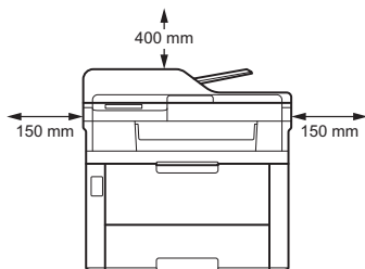
Visão frontal
