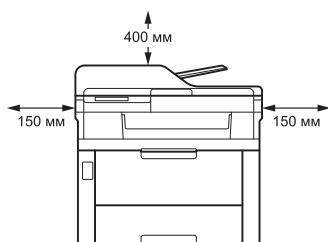
Изглед отпред
