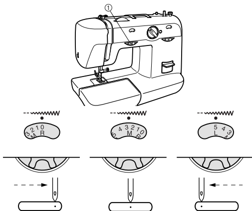
① Stichbreiten-Einstellrad
