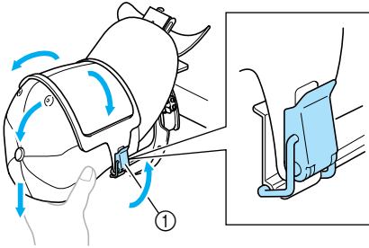
① Hebel des Schnappschlusses
