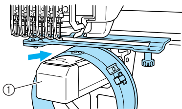
① Maschinenbett
