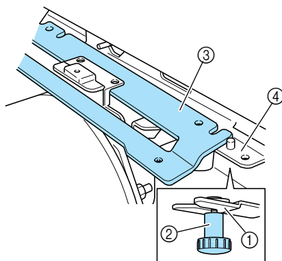
① Kerbe am Stickarm ② Schraube des Kappenrahmenantriebs ③ Montageplatte des Kappenrahmenantriebs ④ Rahmenmontageplatte des Stickarms
