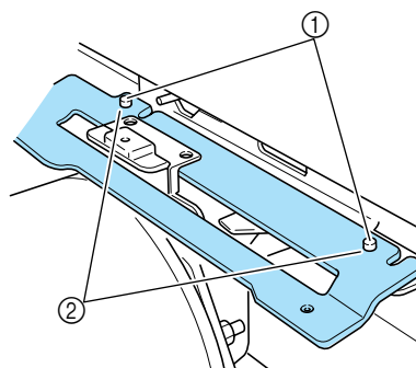
① Stifte an der Rahmenmontageplatte des Stickarms ② Löcher in der Montageplatte des Kappenrahmenantriebs
