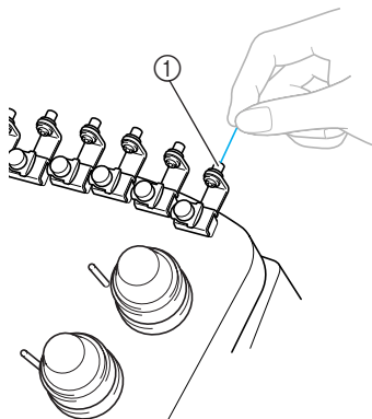
① Trou du guide-fil supérieur
