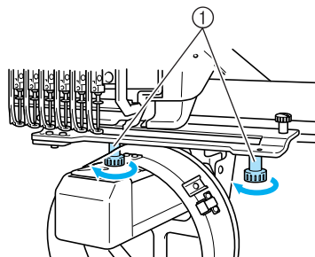
① Vis à serrage à main
