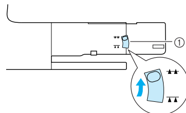
① Transporteur-Einstellhebel
