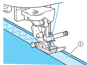
① Gummiband
