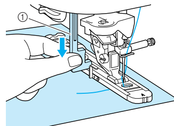
① Knopflochhebel
