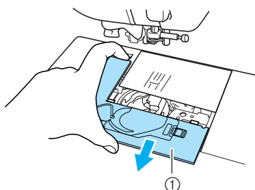
① Stichplattenabdeckung
