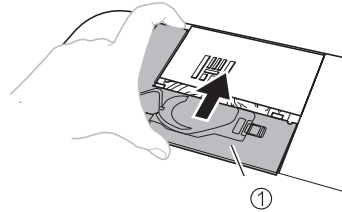
① 針板蓋
