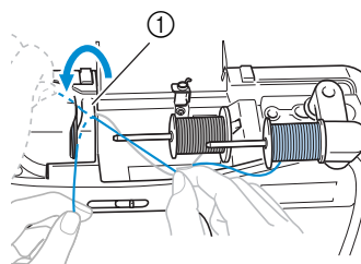
① Крышка направляющей нити
