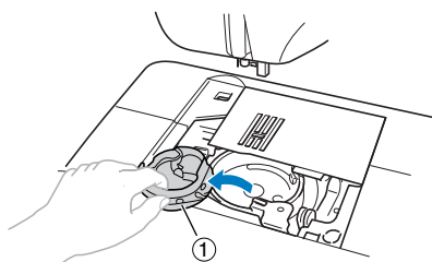
① Caja de la bobina
