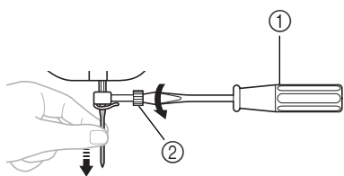
① Cacciavite ② Vite morsetto ago
