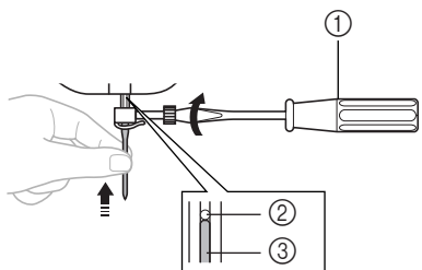
① Cacciavite ② Arresto per ago ③ Ago
