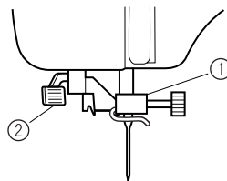
① Supporto dell'ago ② Leva dell'infila ago
