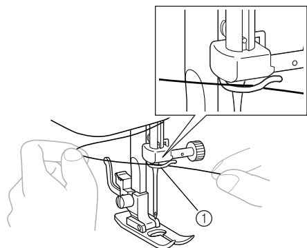
① Guidafile della barra dell'ago
