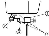
① Supporto dell'ago ② Leva dell'infilo ago ③ Supporto gancio ④ Allineare
