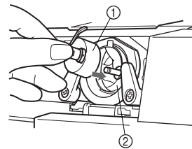
① Compartiment à canette ② Navette
