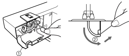
① Couvercle de la navette ② Rainure
