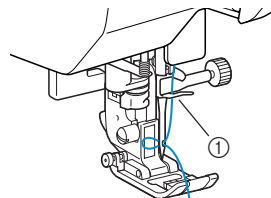
① Направляющий крючок на игловодителе
