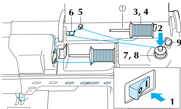
① Lisälankatappi
