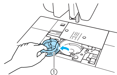
① Puolakotelo
