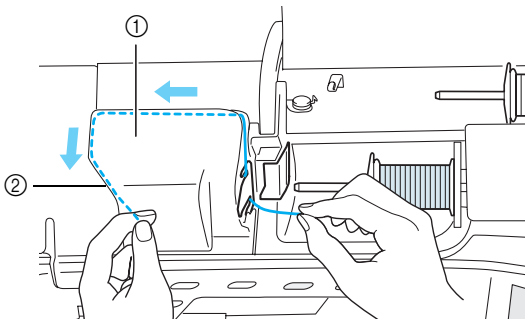
① Pujotusreitin kansi ② Pujotusreitin ohjain
