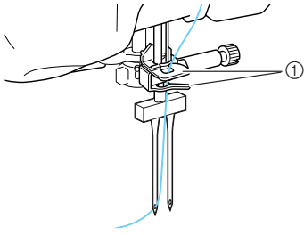
① Neulatangon langanohjaimet
