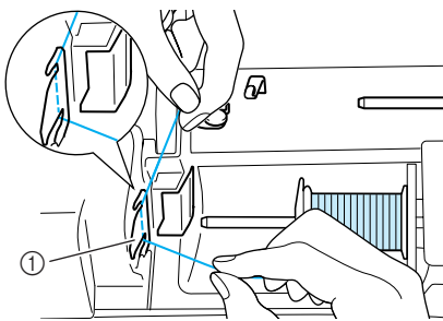
① Langanohjainlevy
