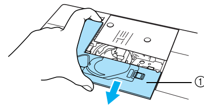
① Pistolevyn kansi
