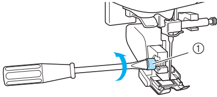
① Tornillo del soporte del pie prensatela
