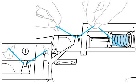
① Fadenführung
