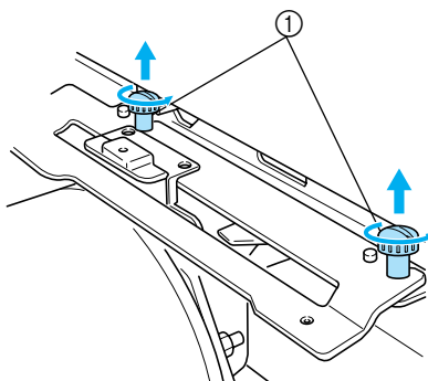
① Винты с накаткой
