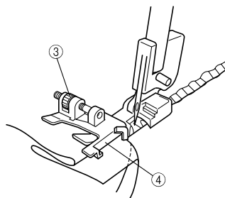
③ Vite di regolazione ④ Guida
