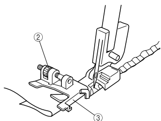
② Vite di regolazione ③ Guida
