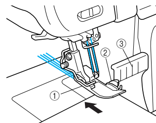
① Nähfuß ② Oberes Messer ③ Materialführung
