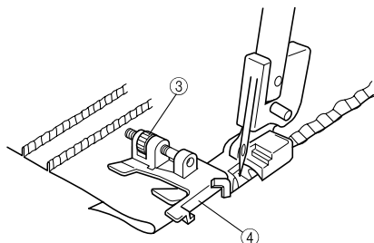
③ Vite di regolazione ④ Guida
