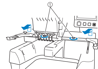
① Tornillos de mariposa
