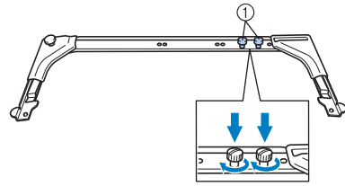
① Vuelva a colocar los dos tornillos de mariposa en el soporte del bastidor.
