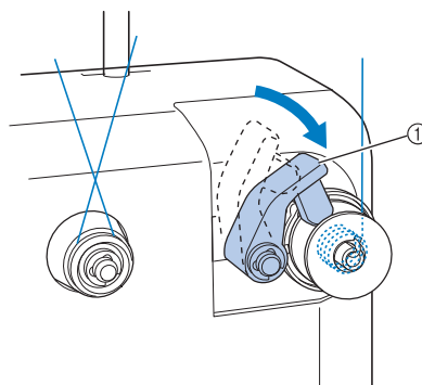
① Soporte de la bobina
