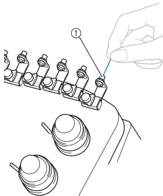
① Foro nel guidafilo superiore
