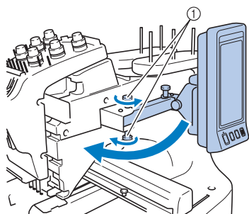
① Viti a testa zigrinata
