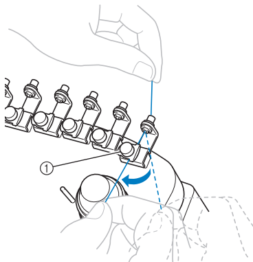
① Guidafilo superiore
