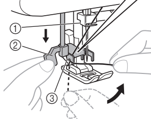
① Nadelhalter ② Nadeleinfädlerhebel ③ Führung
