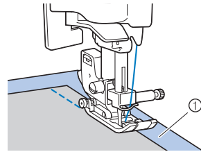
① 종이 또는 보강재
