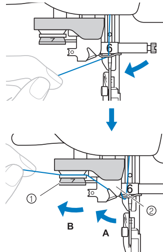
① 실 가이드 디스크 ② 실 가이드
