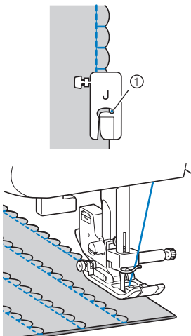
① 바늘이 꿰히는 자리
