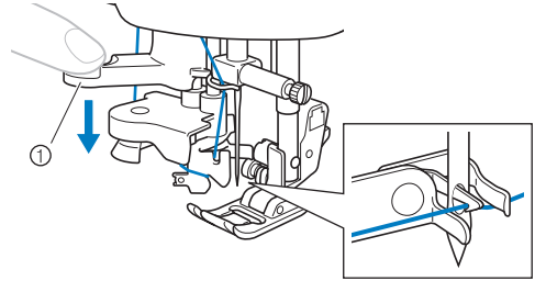
① 자동 실궤기 레버
