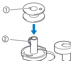
① Muesca ② Resorte del eje de la devanadora de bobina
