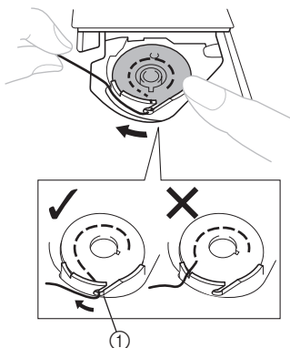
① Ressort de réglage de tension
