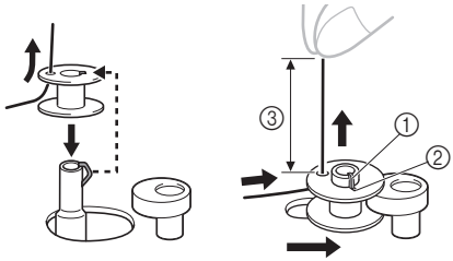
1 Ressort sur l’axe 2 Encoche 3 7-10 cm (3-4 po)
