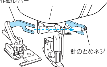
作動レバー
