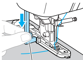
ボタン穴かがりレバー
