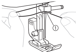
① 바늘대 실 가이드
