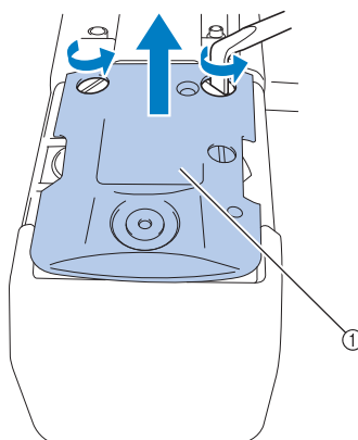
① 針板
