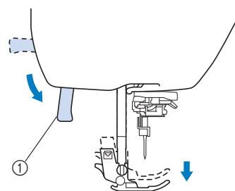
① Nähfußhebel
