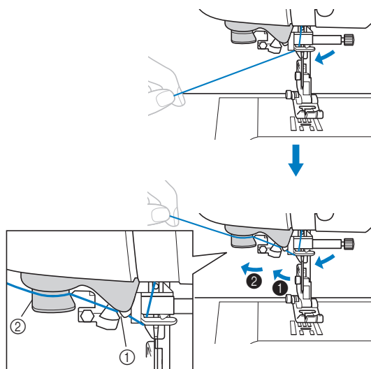
① Kerbe in der Nadeleinfädler-Fadenführung ② Nadeleinfädler-Fadenführungsscheibe
