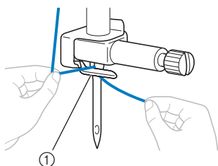
① Fadenführung an der Nadelstange
