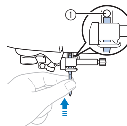
① Nadelanschlag
