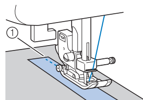
① Bordo del nastro per chiusura velcro
