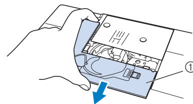
① 針板蓋
