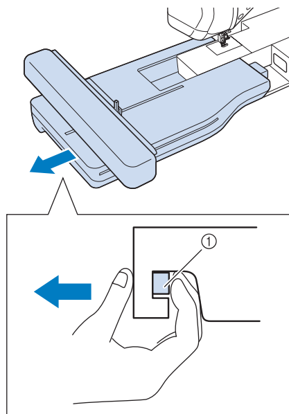
① 鬆開鈕
