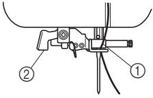
① 바늘 홀더 ② 자동 실 끼우기 장치 레버
