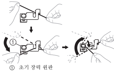
1 초기 장력 원판 2 밀실 감기 장치 축 3 실토리
