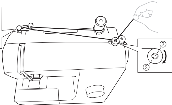
1 초기 장력 원판 2 밀실 감기 장치 축 3 실토리
