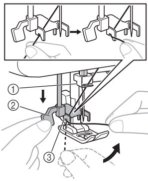
① 바늘 홀더 ② 자동 실 끼우기 장치 레버 ③ 가이드
